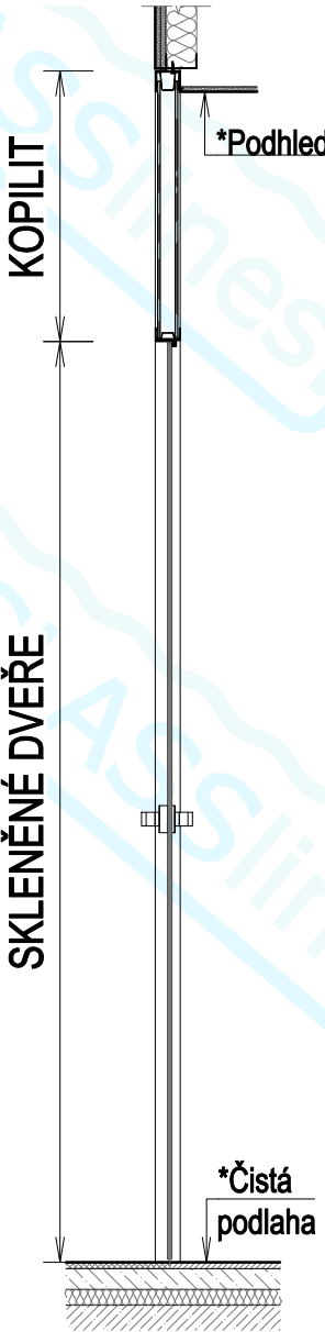
Řez V2 (1:20)
