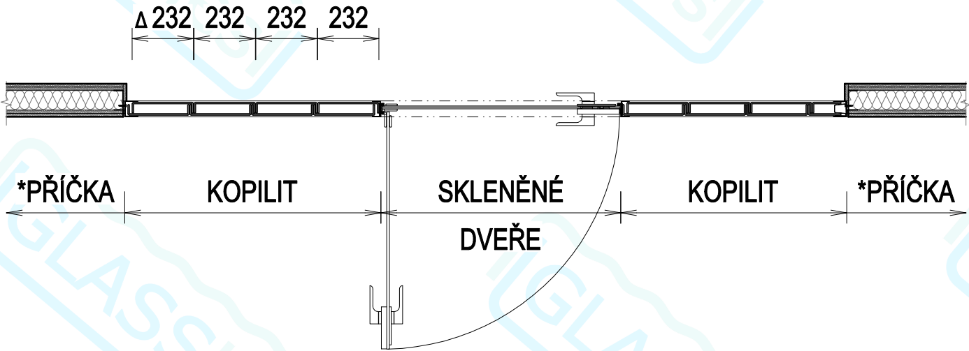
Řez H1 (1:20)
